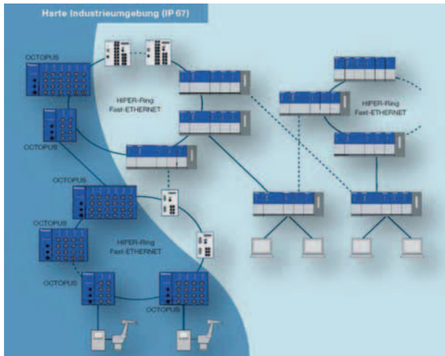
Рис. 8а. Пример построения сети на коммутаторах Hirschmann с использованием технологии кольцевого резервирования Hiper Ring
