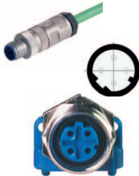
Рис. 7б. Разъём для коммутаторов ОКТОПУС фирмы Hirschmann Electronics
